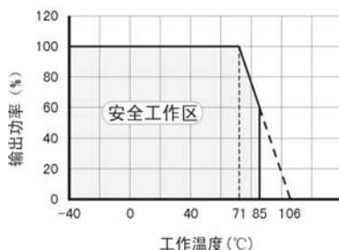
降额曲线图
