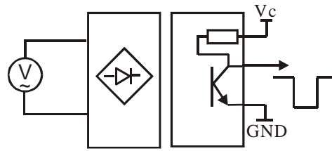
脉冲信号输出
