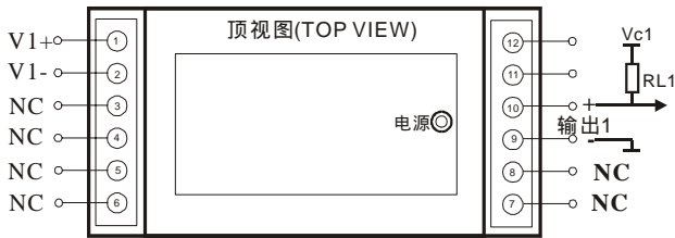
OC 门输出参考接线图
