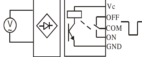
继电器输出
