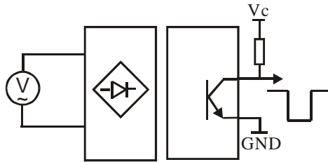
OC 门输出
