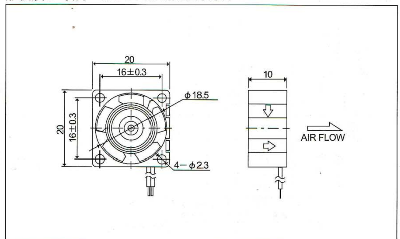
形状及び寸法 SHAPE&DIMENSION
