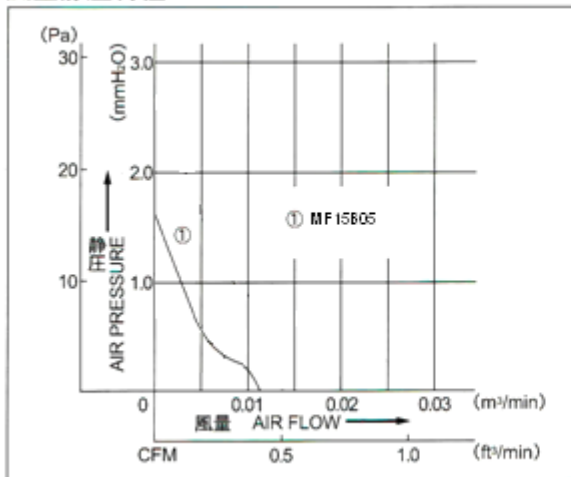
風量静压特性 AIR FLOW VS AIR PRESSURE
