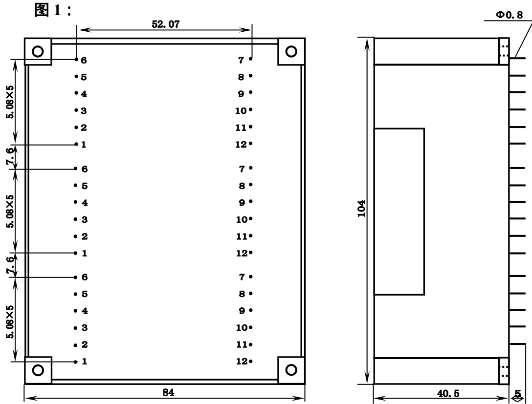
外形背视图
