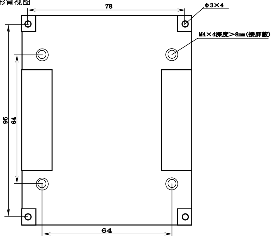
外形背视图
