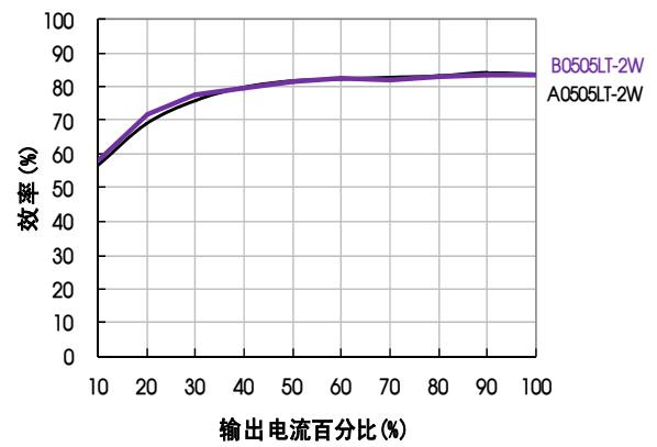
效率Vs输出负载 (标称输入)
