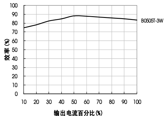
效率Vs输出负载 (标称输入)
