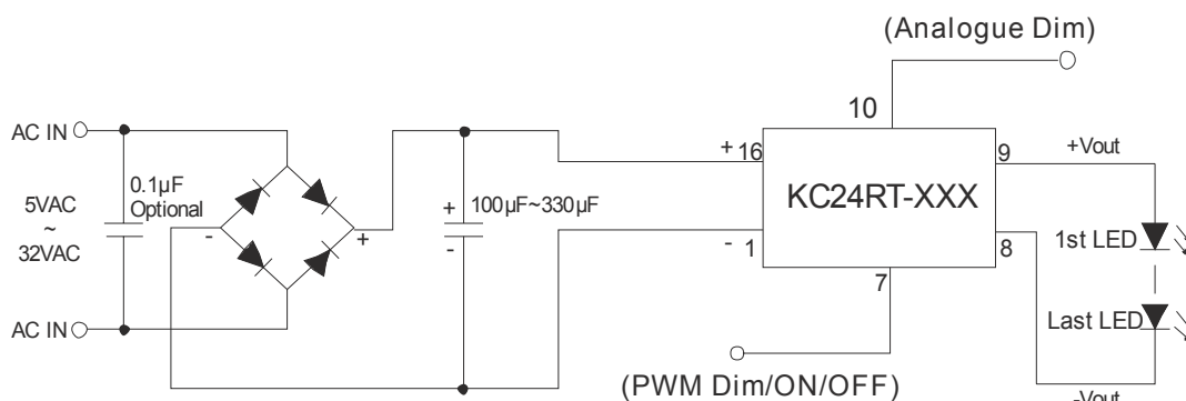
(图 7) AC 输入推荐电路
