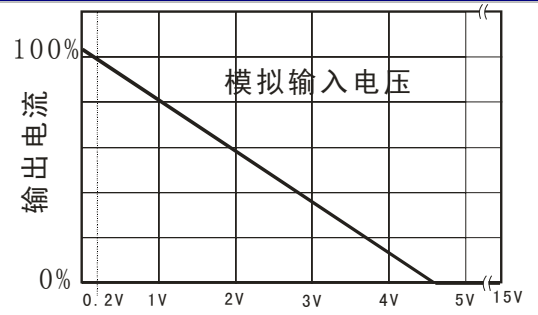
电压控制 (0-15V max) (图 4) 模拟输入电压与输出关系
