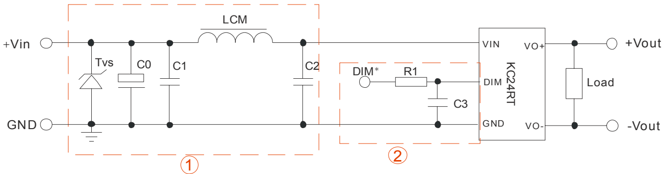
(图 6) EMI/EMC 推荐电路
