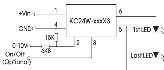
(图 8) 模拟调光电路
