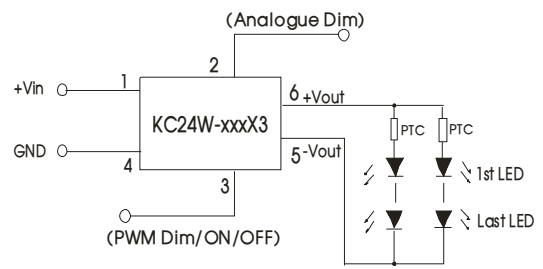
图 3 串并联应用
