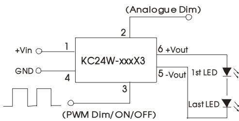
图 2 串联应用
