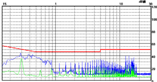
WRB2405MT-3W 传导骚扰 Class B 测试效果图（正线）
