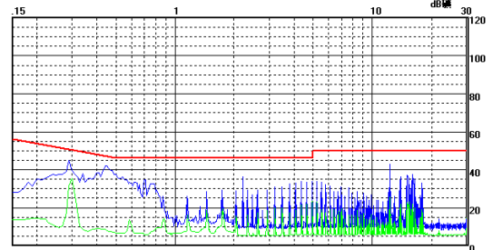
WRB2405MT-3W 传导骚扰 Class B 测试效果图（负线）
