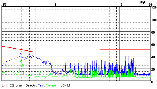
WRF2405MT-3W 传导骚扰 Class B 测试效果图 (正线)
