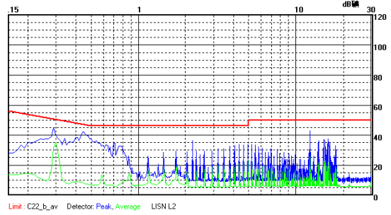
WRF2405MT-3W 传导骚扰 Class B 测试效果图 (负线)
