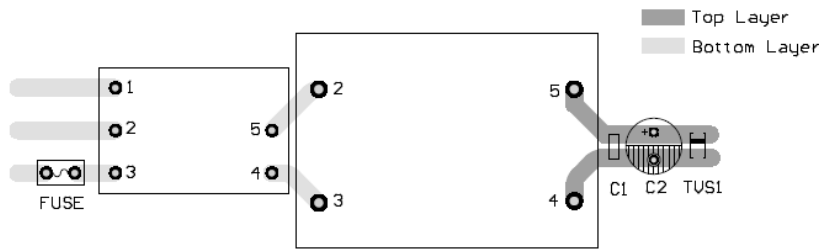
图 3:EMC 推荐电路 PCB 布板图 常规及走线宽度建议: 线宽 ≥3mm, 线线距离 ≥6mm, 线地距离 ≥6mm
