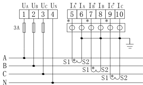
三相四线3CT
