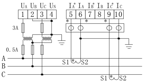
三相三线2PT、2CT
