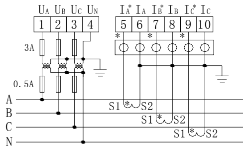
三相四线3PT、3CT
