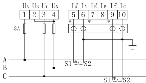
三相三线2CT
